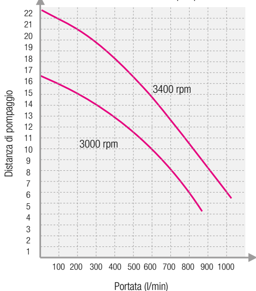
Curva caratteristica della pompa
